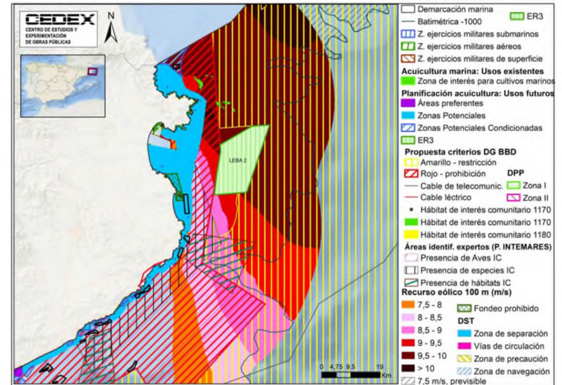
Figura 271. Delimitació de los polígonos ER3 para el desarrollo de la eólica marina en la Demarcación levantino-balear. Solape con todos los usos y actividades en la demarcación. Detalle del polígono LEBA 2 (Fuente: Elaboración propia)
