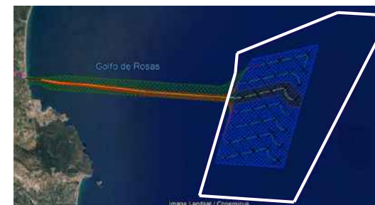
Figura 271. Delimitació de los polígonos ER3 para el desarrollo de la eólica marina en la Demarcación levantino-balear. Solape con todos los usos y actividades en la demarcación. Detalle del polígono LEBA 2 (Fuente: Elaboración propia)
